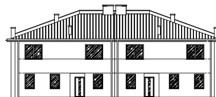
ELEWACJA FRONTOWA
