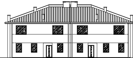
ELEWACJA FRONTOWA
